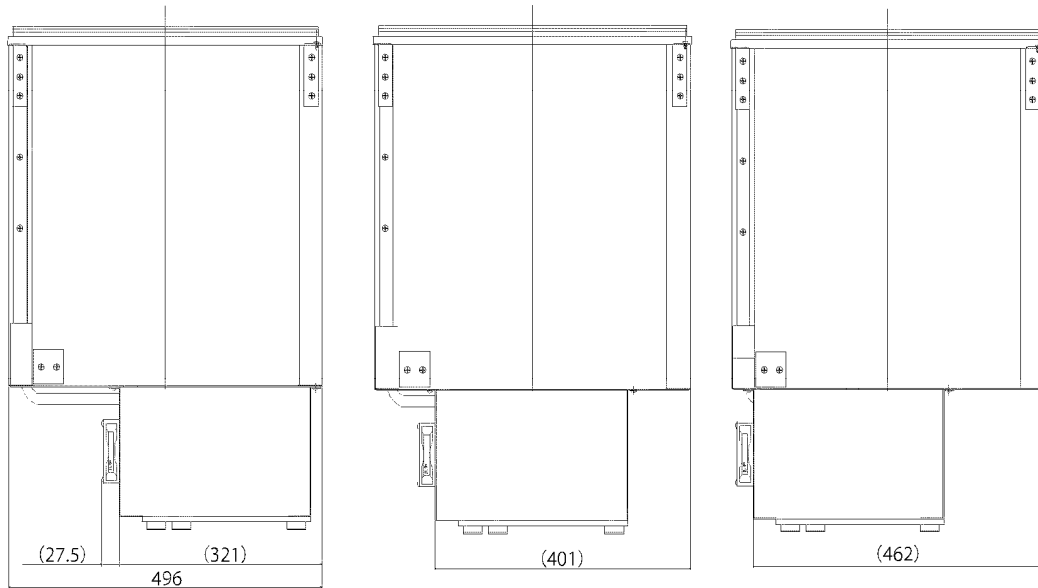
①機械部の位置が冷蔵庫の右側 (ご購入時の状態)
