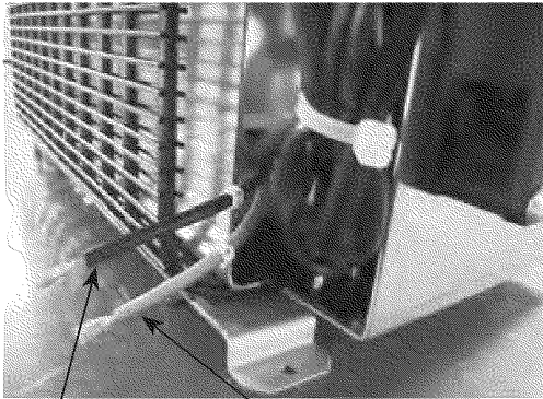
⊖ マイナス側 (黒) ⊕ プラス側 (赤)
