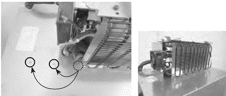
例) ②の位置(冷蔵庫のほぼ中央) に固定した場合
